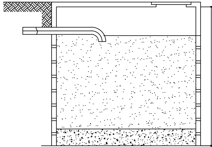
Sumidouro - Corte Esc. 1:50
