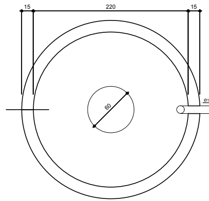
Tanque Séptico - Planta Baixa Esc. 1:50
