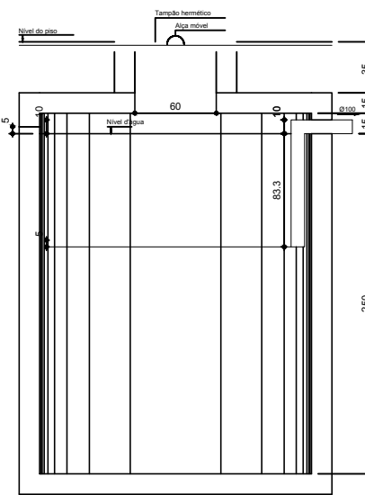
Tanque Séptico - Corte Esc. 1:50
