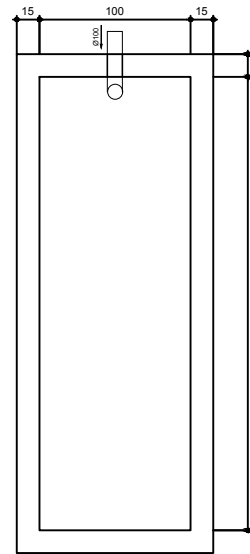
Sumidouro - Planta Baixa Esc. 1:50
